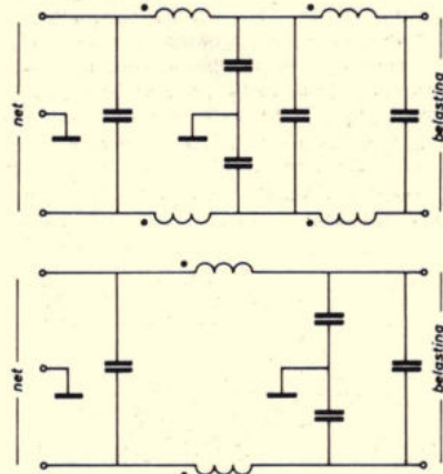
Fig. 1. Het bovenste schema toont twee T-sectie filters voor onderdrukking van asymmetrische RFI storing. Dit filter is bijzonder effectief, wanneer de belasting een lage impedantie heeft, zoals een motor.
